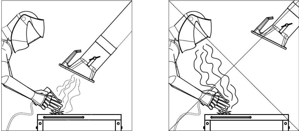
Fig. 6: Posizionamento della cappa di aspirazione
