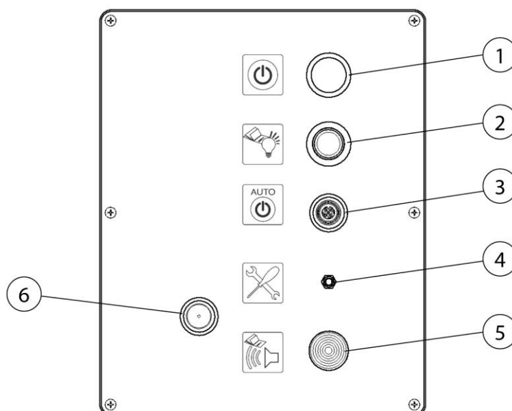
Fig. 5: Elementi di comando
