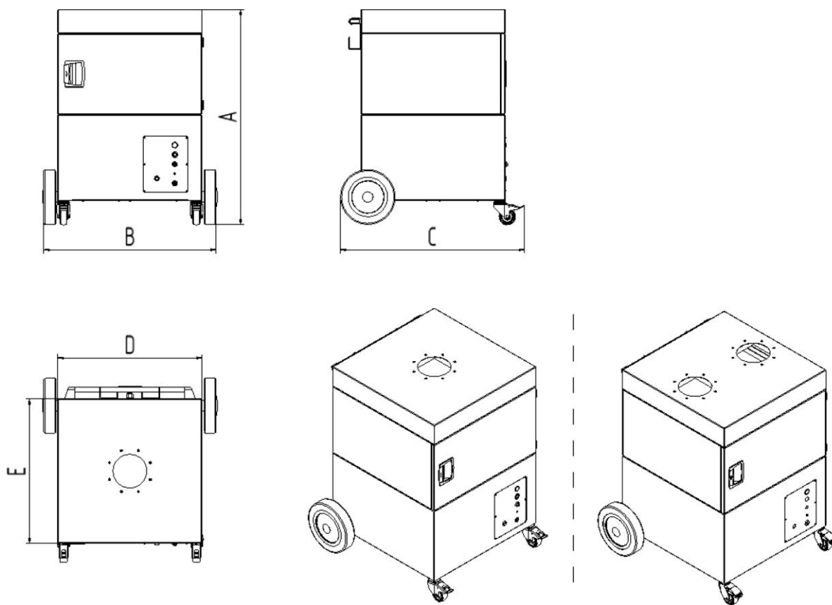
Fig. 9: Disegno quotato 60650 + 60650DA
